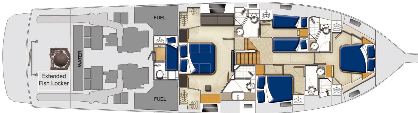
Optional crew cabin
